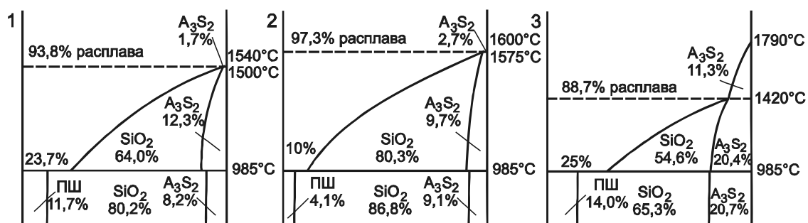
Рис. 1. Диаграммы плавления песков Краматорского (1), Райского (2) и Дружковского участков (3)
